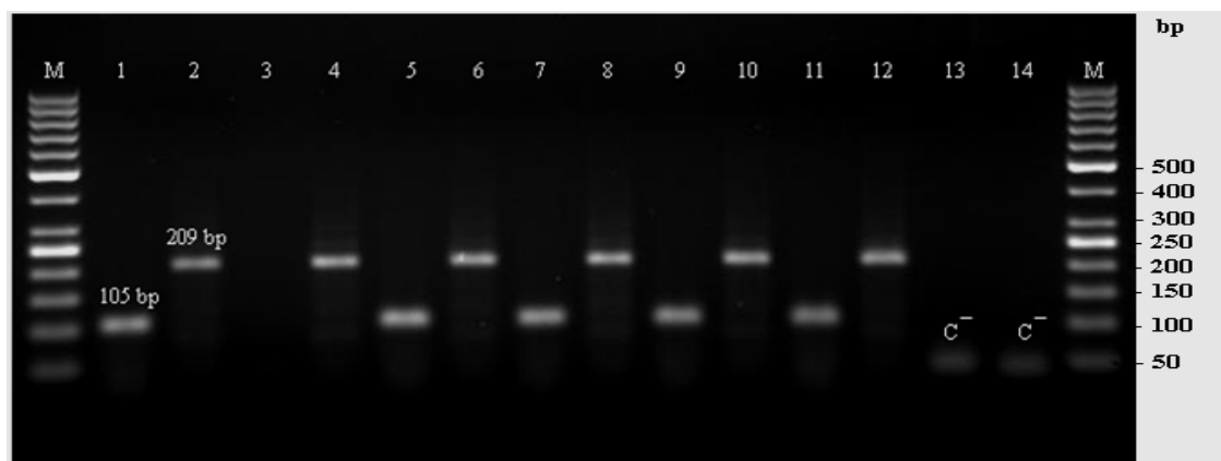
تصویر ۱: نتایج حاصل از الکتروفورز محصول واکنش زنجیره ای پلی‌مراز معکوس ژن های ACT1 و CDR2
