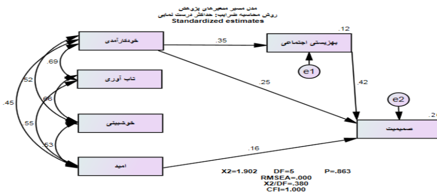
مدل ۱: تحلیل مسیر مدل تأثیر سرمایه‌های روانشناختی با نقش واسطه‌ای بهزیستی اجتماعی بر صمیمیت زناشویی (روش محاسبه ضرایب: حداکثر درست نمایی)
